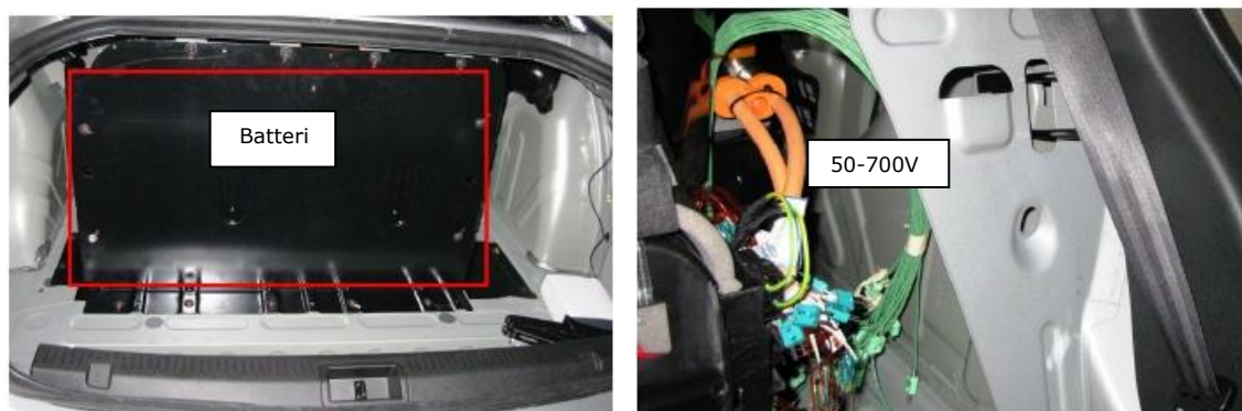
Til venstre ses batteriet fra et åbent bagagerum. Til højre ses ledningsnettet bagved passagersædet i el-køretøjet.
