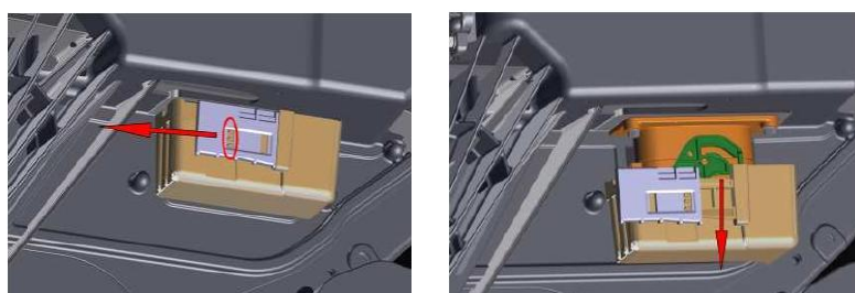
Afmontering af beskyttelsesdæksel til sikkerhedsafbryder.
