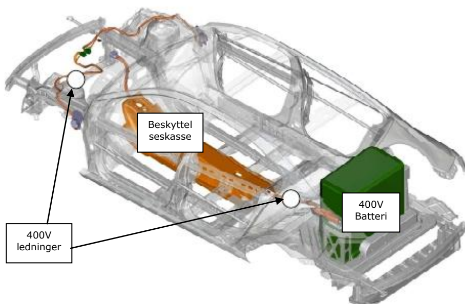
Et eksempel på et 400 volt batteri placeret bag bagsæderne på en Renault Fluence med 400 V ledninger ført i en beskyttelseskasse.
