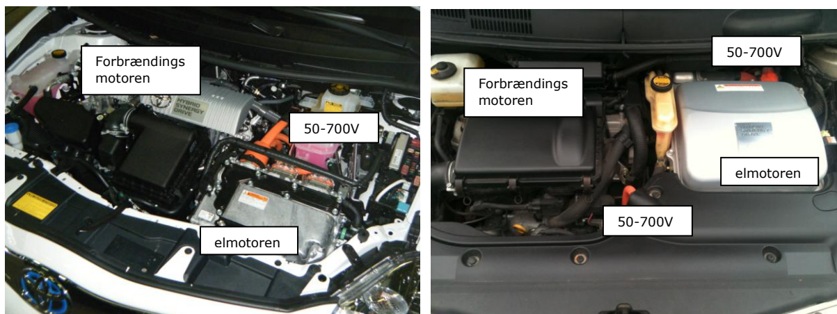
Motorrum på et hybridkøretøj med forbrændingsmotor og el-motor.
